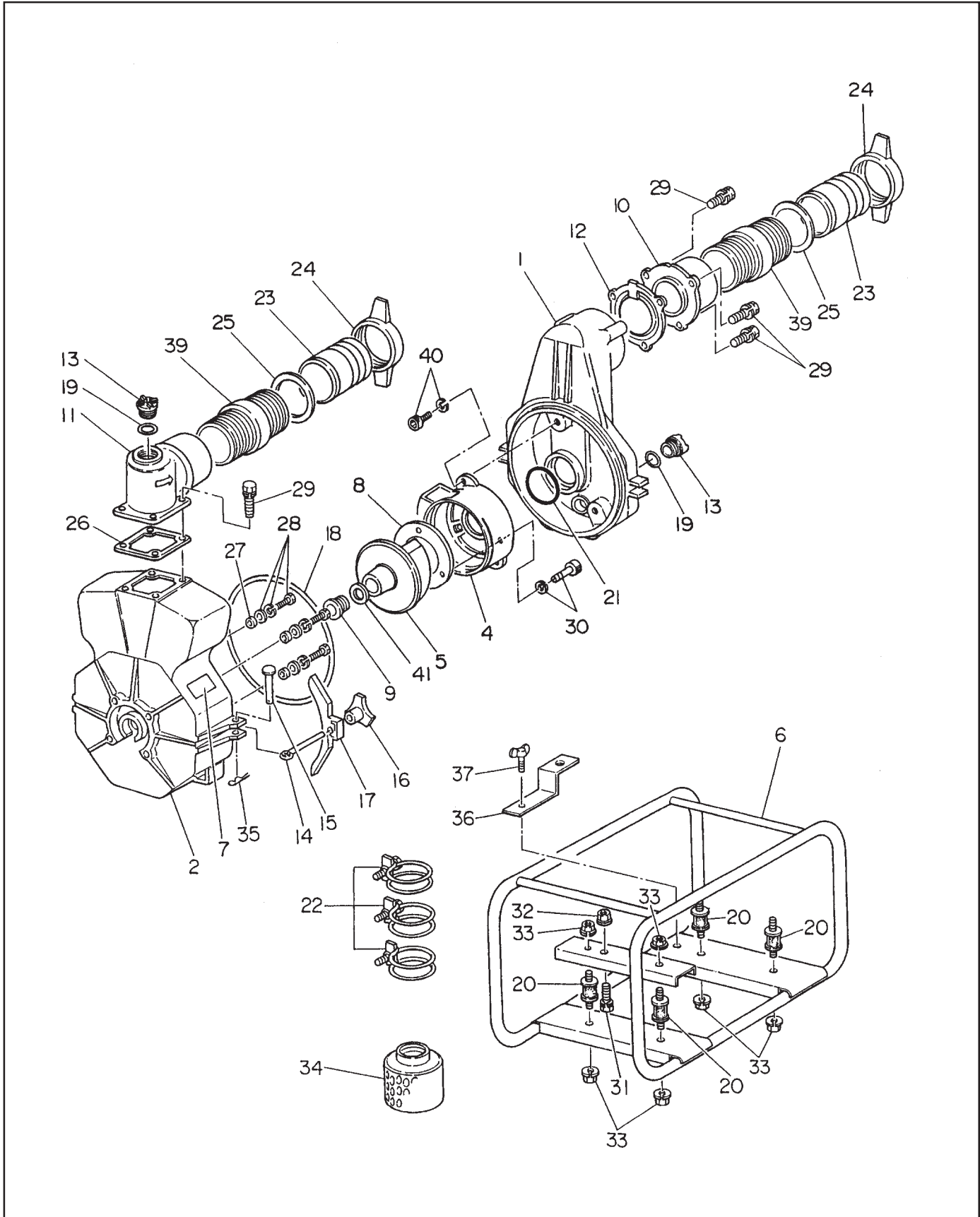
FIG. 1A PUMP - PTD206T
