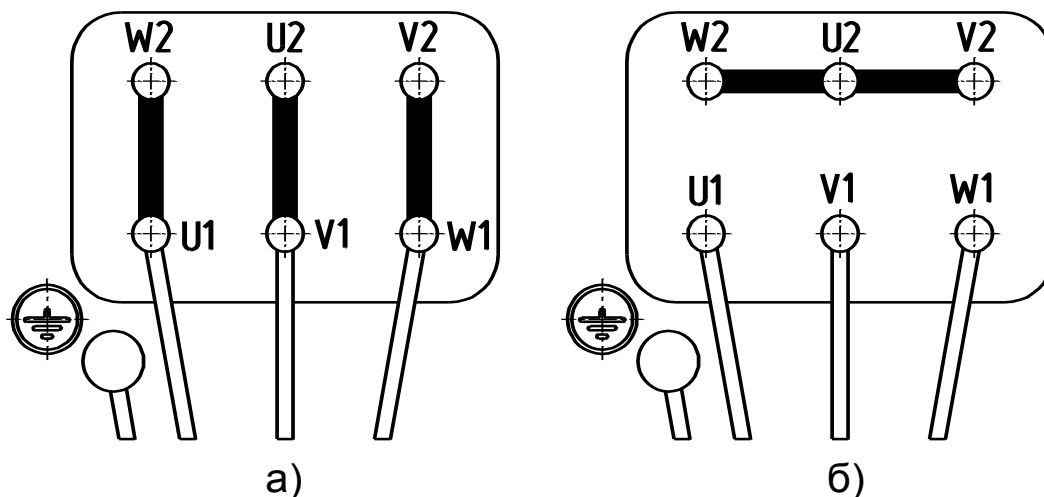
Рисунок 3. Схема соединения обмоток статора:
