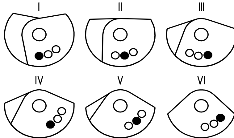
Рисунок 4. Схема регулировки статического момента ступенчато регулируемых дебалансов вибраторов ИВ–11-50, ИВ–11-50Н, ИВ- 98Н, ИВ–06-25, ИВ–06-25Н и ИВ–104Н.
