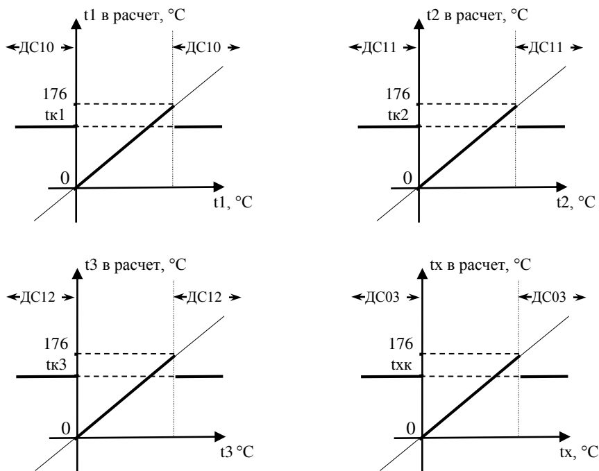
Рисунок 6.3 – Контроль температуры и использование констант
