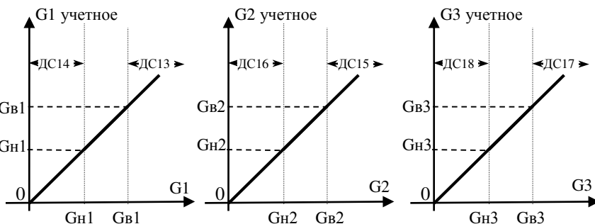
Рисунок 6.2 – Контроль объемного расхода при KG=0
