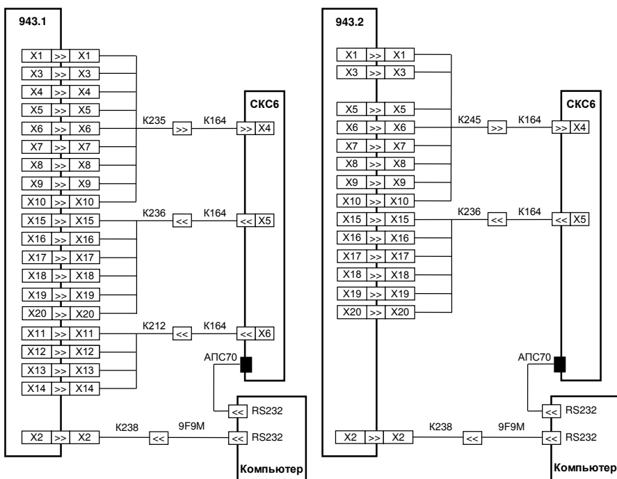
Рисунок 5.1 – Схемы поверки
