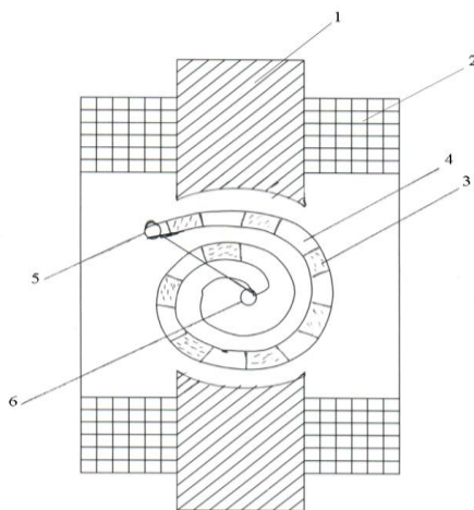
Рисунок 1. Конструкция СВ: 1-индуктор; 2-обмотка статора; 3-спиральная пружина; 4-прорези продольные со скосом; 5,6-валы СВ
