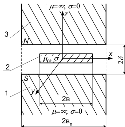
Рисунок 2. Расчетная схема: 1; 3-индуктор; 2-виток спирали с продольными косыми прорезями.
