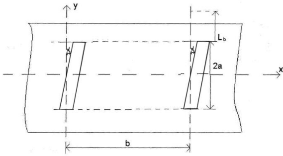
Рисунок 3. Спиральный виток с косыми прорезями.
