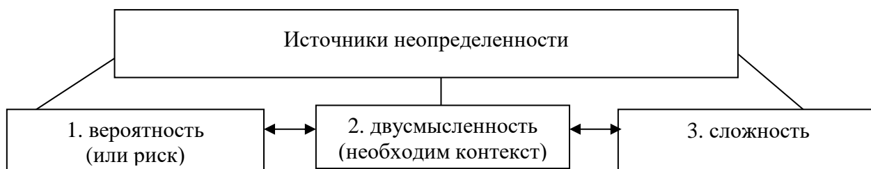
Рисунок 1. Источники неопределенности
