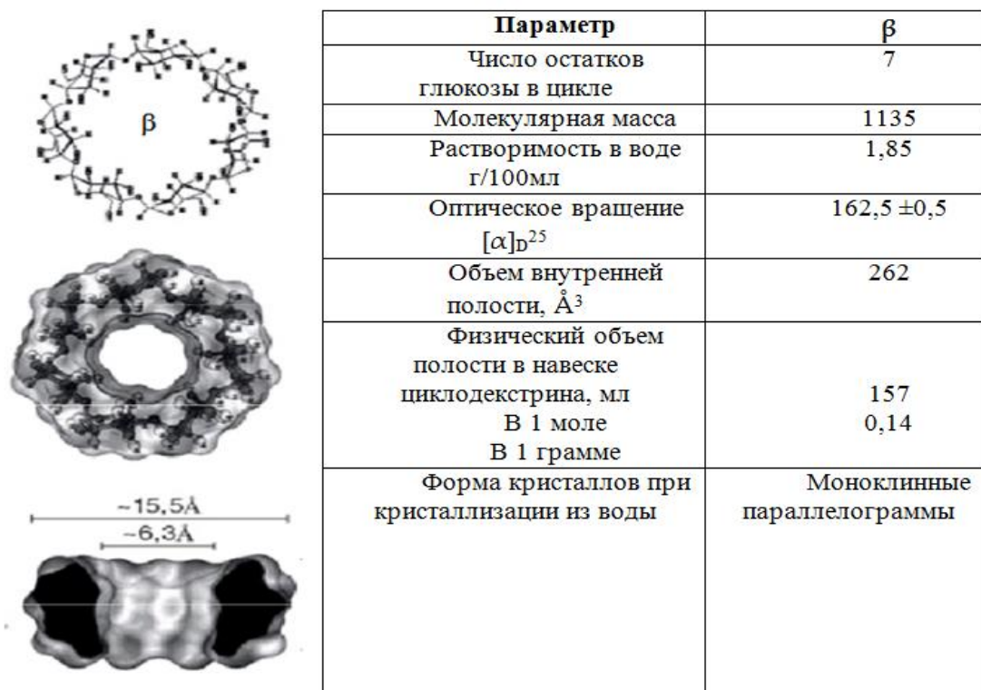
Рисунок 1. Свойства и структурная модель \beta -циклодекстрина [4]
