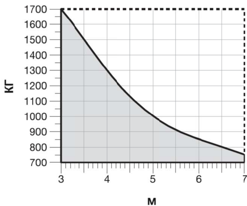
График 2 Привод Тоона 4
