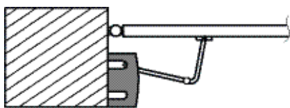
Монтаж на колонну, открытие наружу
