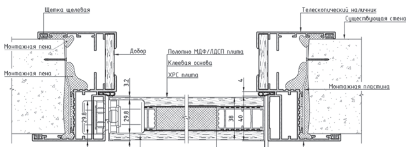
Схема внутреннего открывания (IN)
