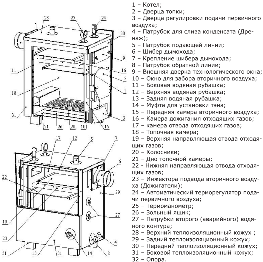
Рисунок 4. Устройство котла серии «Т»
