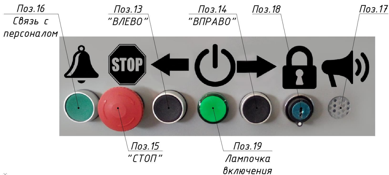
Рисунок 4 Устройство управления подъемной платформой
