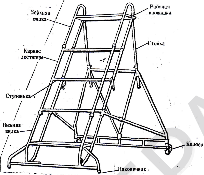
Стремянка АЗ8-0100-0
