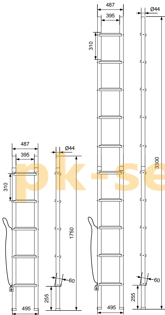
Рисунок 1. Габаритные размеры (одно звено)
