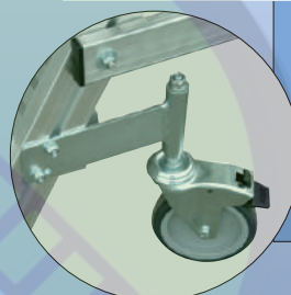
4 поворотных ролика ( \varnothing 125 мм), стопорящихся при подъеме по лестнице, 2 со стояночным тормозом
