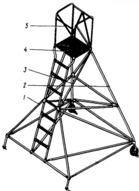
Рис. 62. Стремянка:
