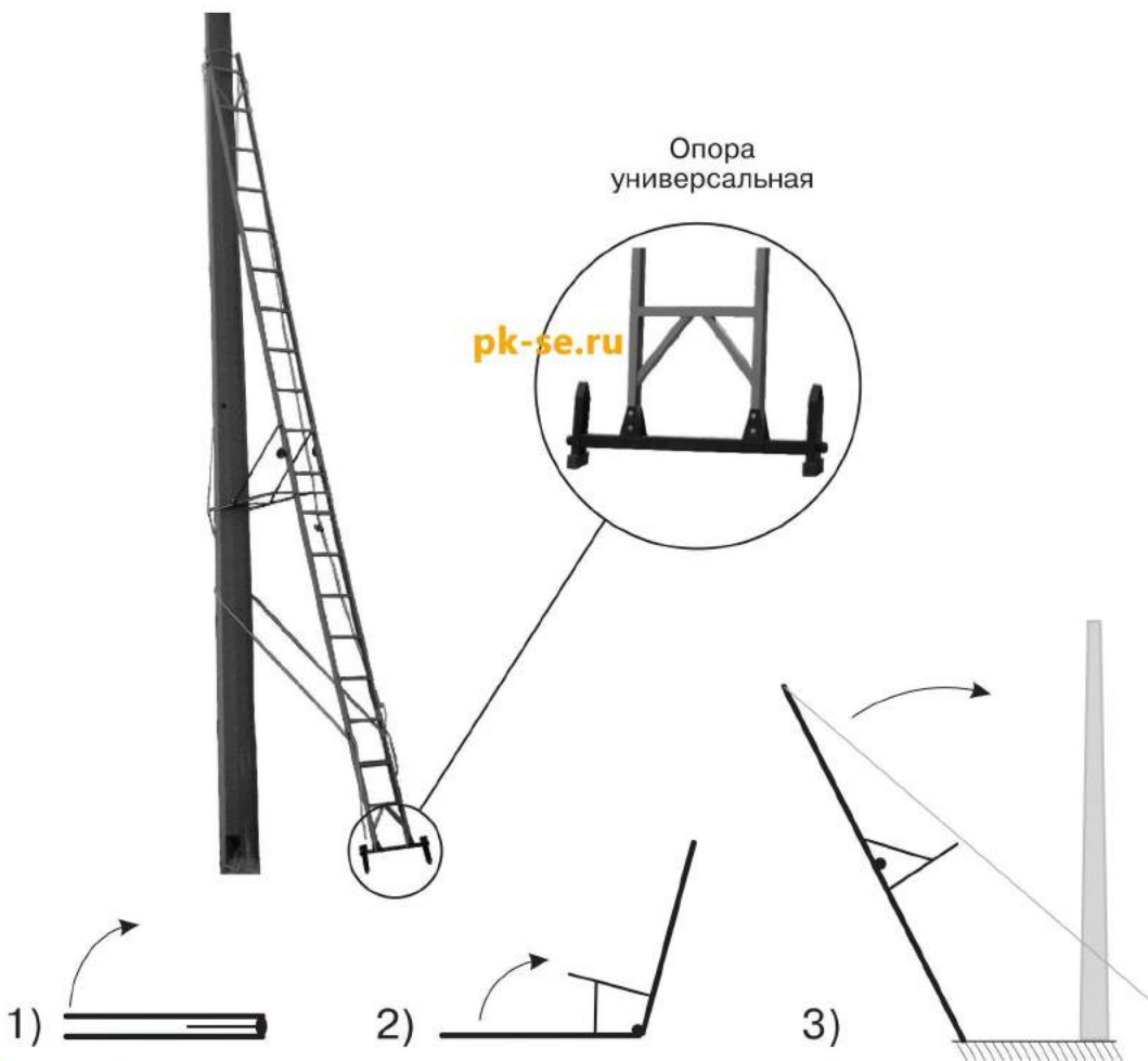
Схема монтажа
