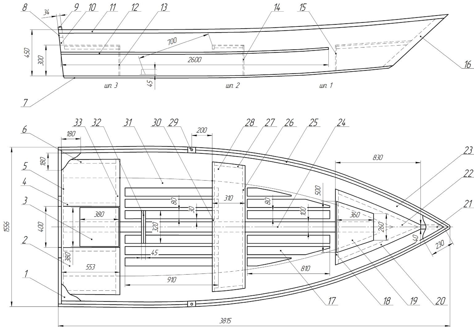
Рис. 9 Конструкционный чертеж моторной лодки “Щука”
