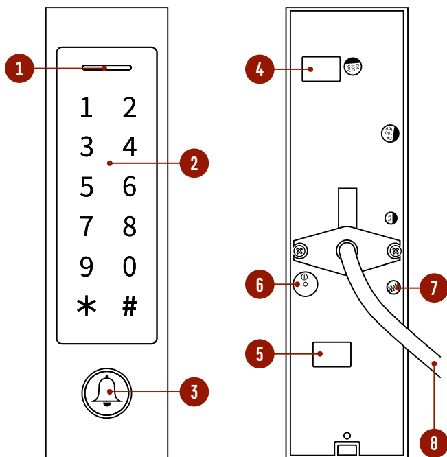
Рис. 2 Описание контроллера SE410KW WIFI
