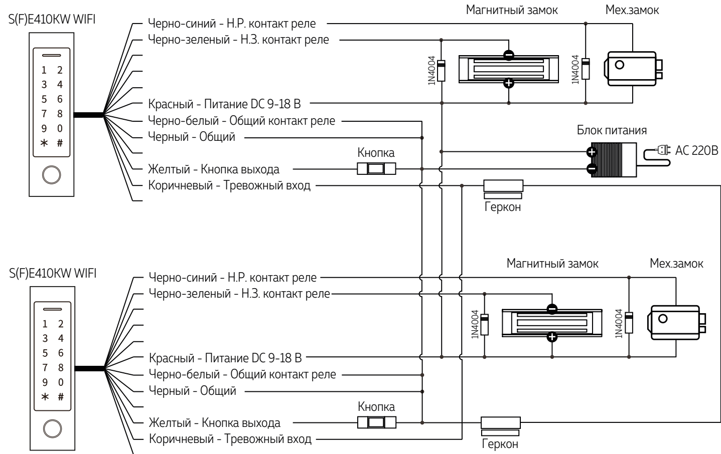
Рис. 9 Схема подключения контроллеров для организации шлюза
