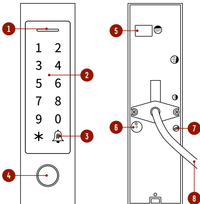
Рис. 3 Описание контроллера SFE410KW WIFI
