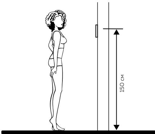
Рис. 7 Рекомендуемая высота установки видеодомофона и вызывной панели
