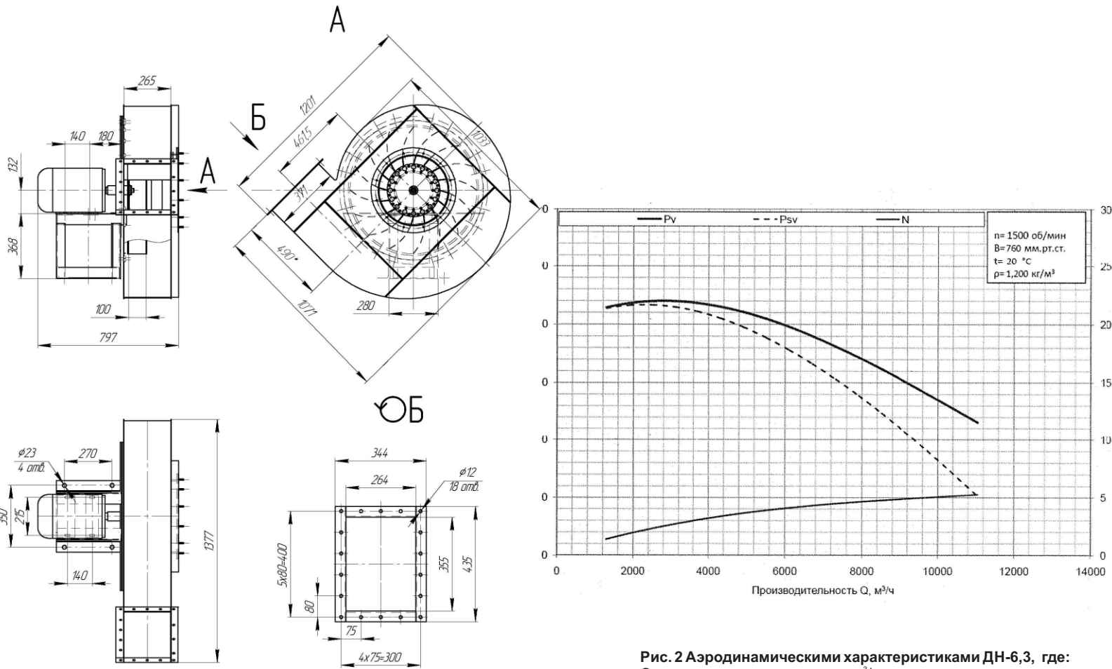
Рис. 2 Аэродинамическими характеристиками ДН-6,3, где: Q — производительность, тыс. м³/час; N- мощность, потребляемая вентилятором (дымососом), кВт; Pv — полное давление, Па; Pdv - динамическое давление, Па; η - коэффициент полезного действия, %; n — частота вращения рабочего колеса, об/мин; Vвх — средняя скорость воздуха в выходном сечении дымососа, м/с.
