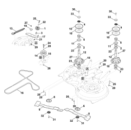
Привод ножа
