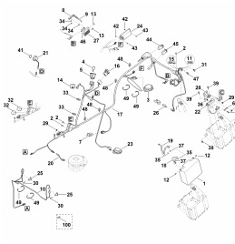
Узлы электрооборудования
