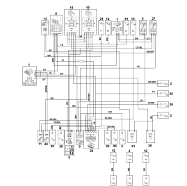
Схема контактов
