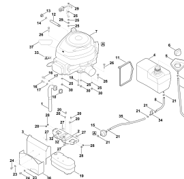
Двигатель, бак
