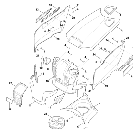
Кожух двигателя
