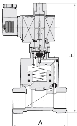
Рисунок 1. Эскиз
