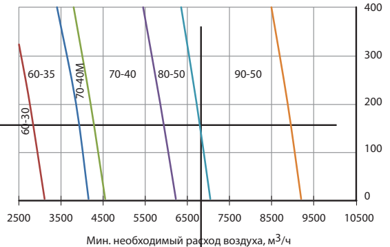
Номограмма 5
