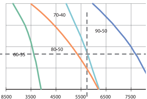
Мин. необходимый расход воздуха, м³/ч
