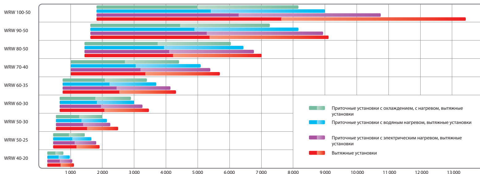
Воздухопроизводительность
