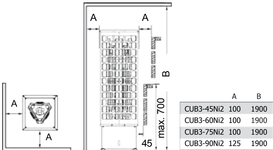
Рис. 2 | Минимальные безопасные расстояния (мм) Fig. 2 | Minimum safety distances (mm)
