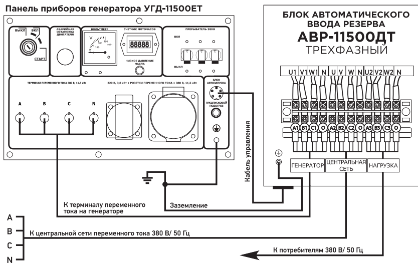
Рис. 13. Схема подключения резерва АВР-11500ДТ
