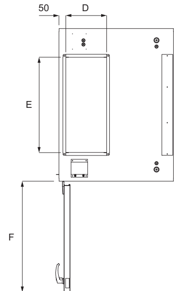
Секция SoftCooler. Вид сверху
