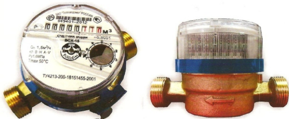
Рис. 9 Счетчик холодной (горячей) воды BCX-15-02R (BCG-15-02R) (предназначены под накладку, используемую для передачи данных по радиоканалу)
