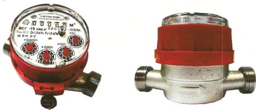
Рис 2. Счетчик горячей воды ВСГ-15
