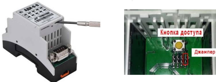
Рисунок 5.1 – Разрешение/запрет конфигурирования
