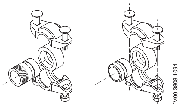
Муфта PJE
