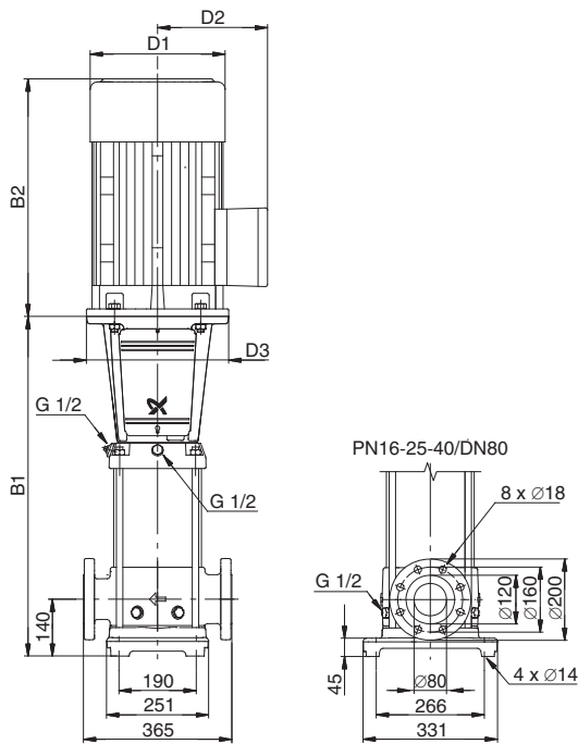
Питательный насос CRN / насос высокого давления CRN
