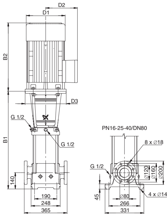
Питательный насос CR / насос высокого давления CR
