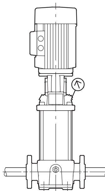
Рис. 34. Уплотнение вала.
