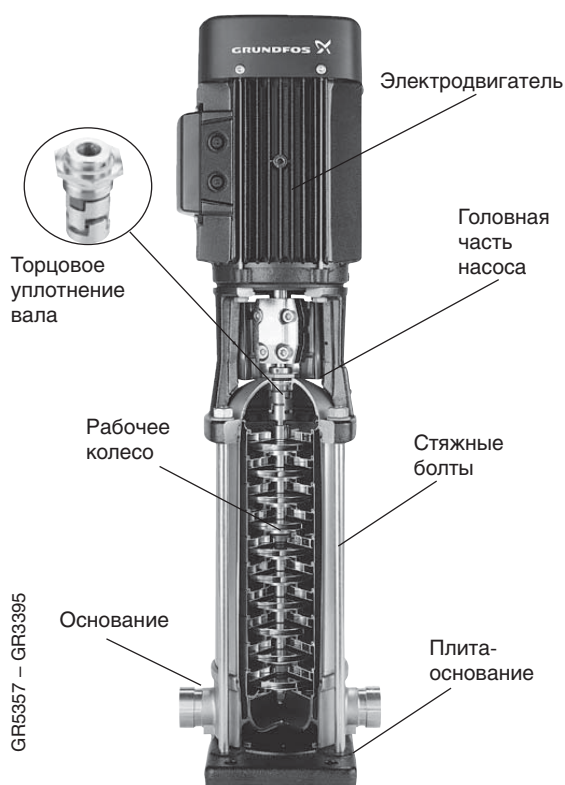
Рис. 3. Насос CR.
