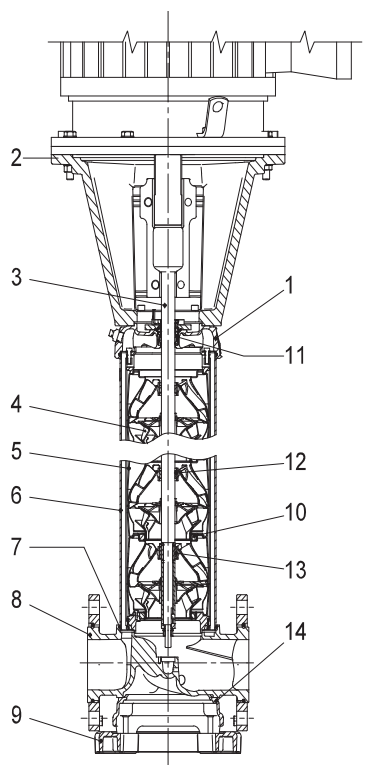
Рис. 42. Чертеж насоса CR(N) в разрезе
