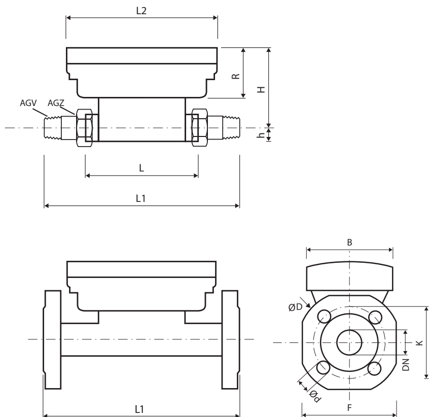
Рис. 1. Габаритные размеры
