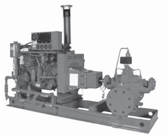
Рис. 31 Внешний вид дизель-насосной установки пожаротушения
