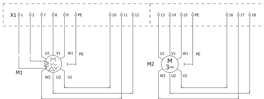
Основной насос
