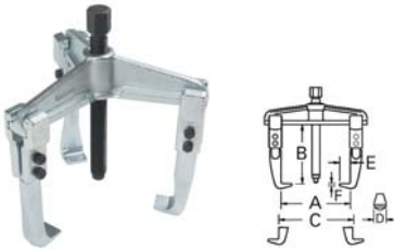
GPL-AS Съемник с тремя передвжными захватами, американский тип
