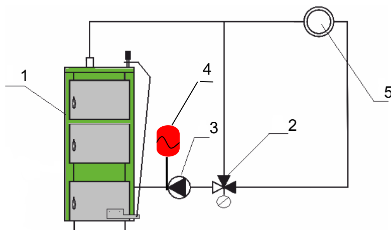
1. Котел на твердом топливе Lavoro серии M 2. Термостатический смесительный клапан 3. Насос ЦО 4. Мембранный расширительный бак 5. Потребители тепла
