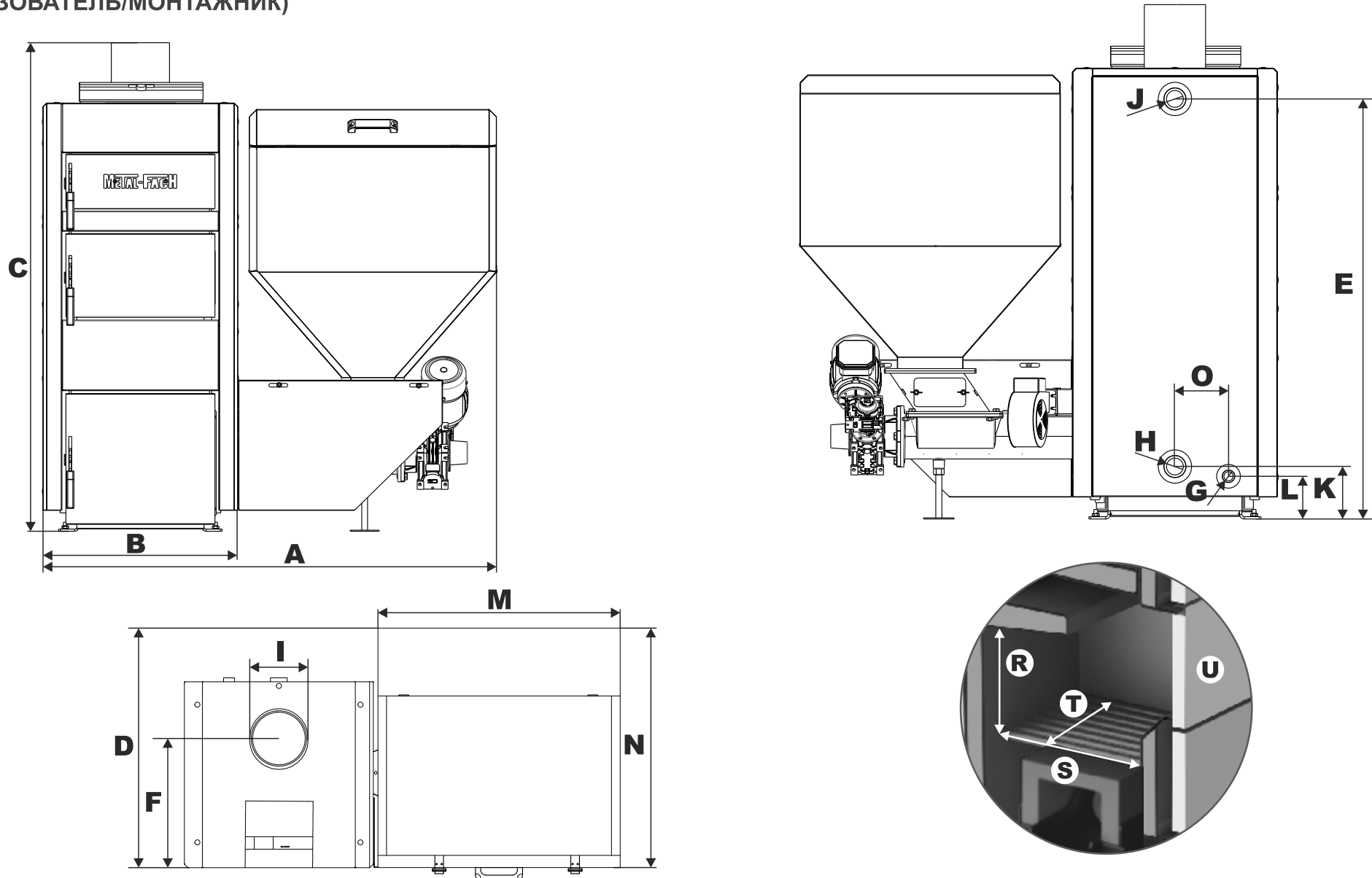
Рисунок 7.4 Размеры котла SMART BIO
