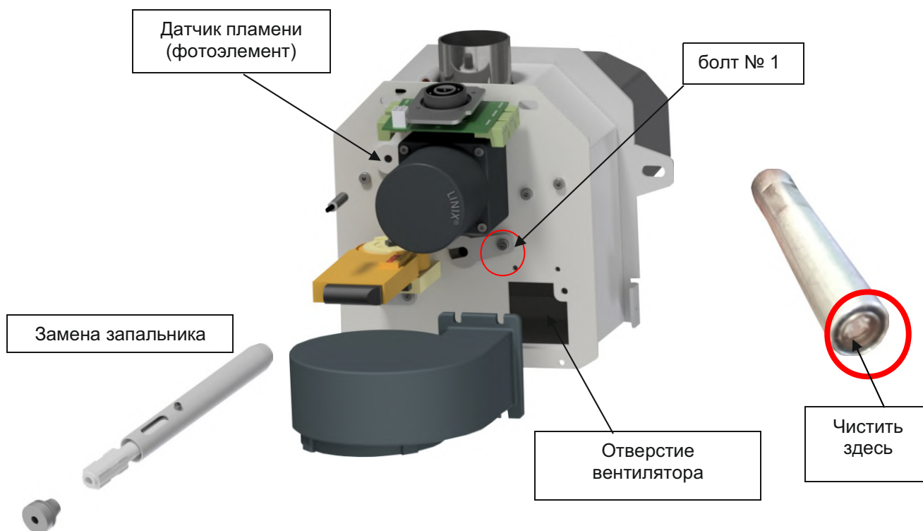
Рисунок 10 - Схема демонтируемых узлов для очистки и ревизии
