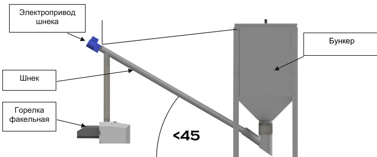
Рисунок 7 – Общий вид винтового подающего устройства с Горелкой и бункером
