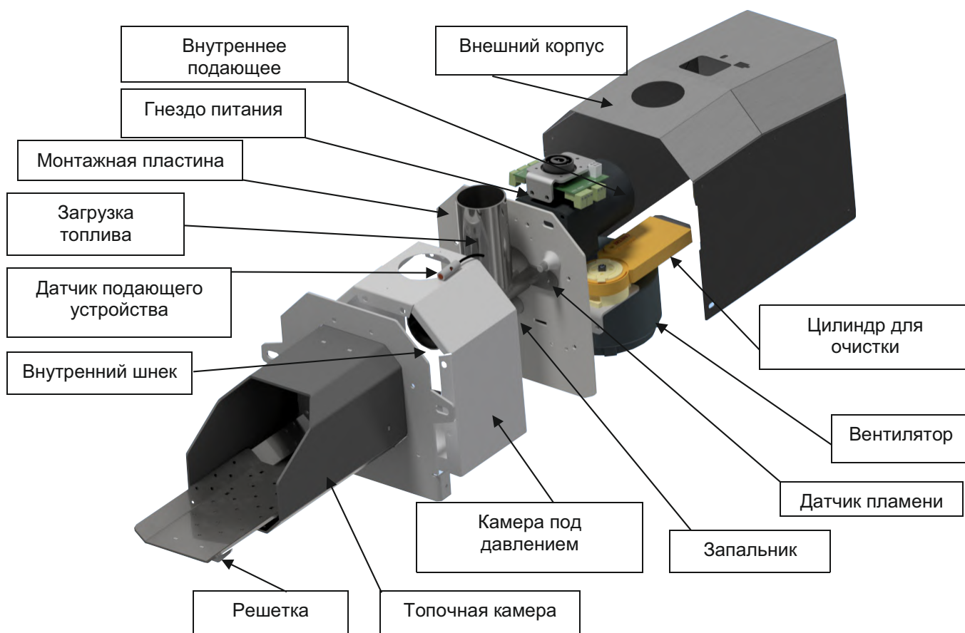
Рисунок 6 – Состав Горелок Lavoego Eco 16-102
