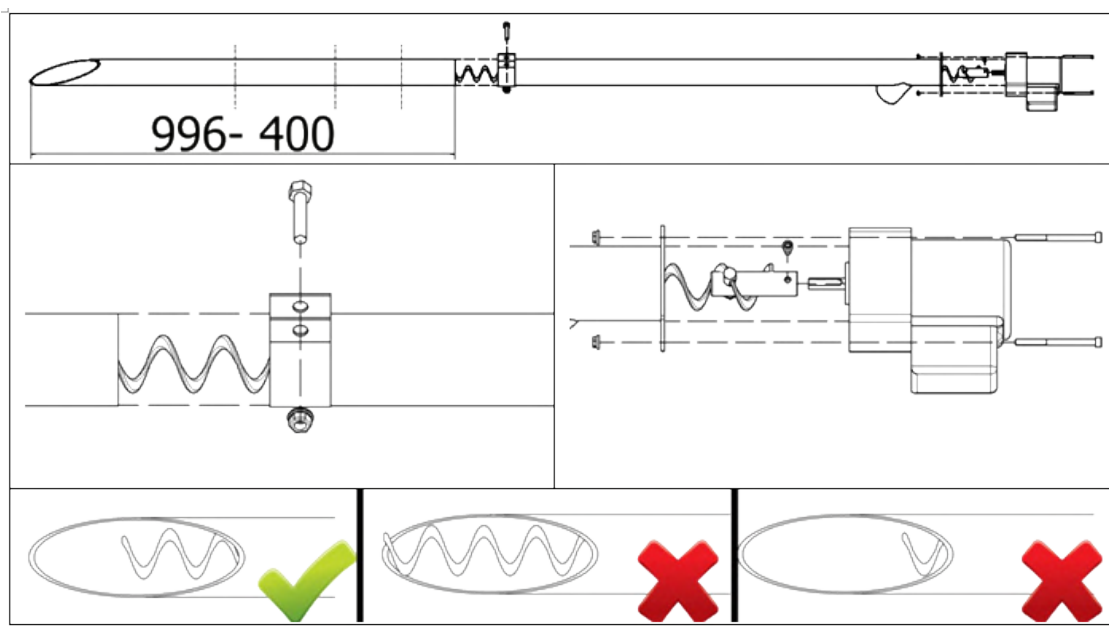
Рисунок 9 – Схема установки винтового подающего устройства в штуцере бункера
