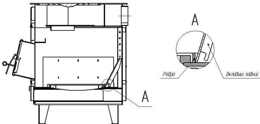
Рисунок 5б - Установка вкладыша заднего в топку печи
