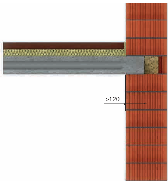
Рис. 13. Опирание плит перекрытия на кладку из блоков Porotherm
