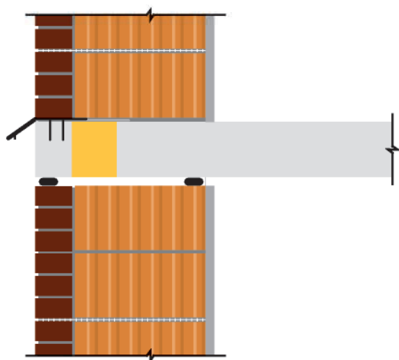
Монолитно-каркасная стена:
