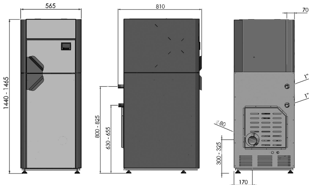
Рис.1. Вид котла
