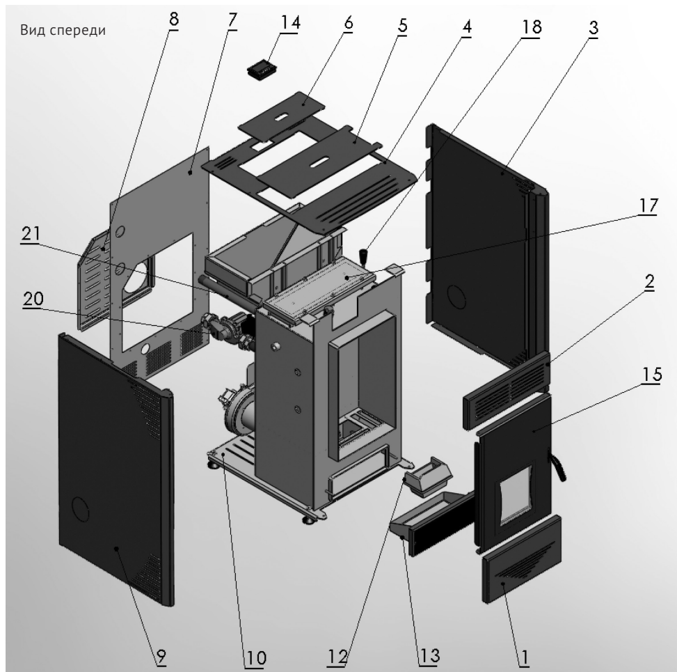
Рис.3. Детали котла TOBY 12 Н
