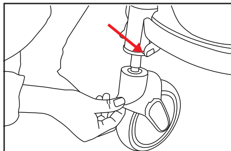
7. Снятие передних колес: нажмите на кнопку, как показано на рисунке и вытащите колесо.
