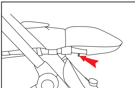
2. Регулировка подножки: нажмите на кнопки, как показано на рисунке, чтобы поднять подножку.
