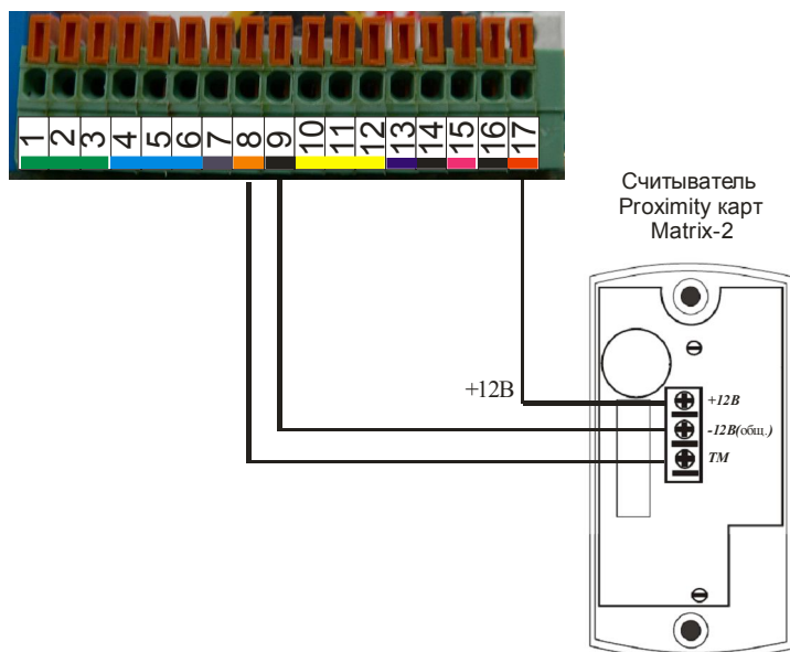
4. Схема подключения различных считывателей ключей.
