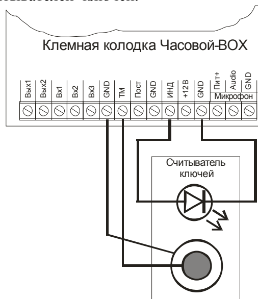
4. Схема подключения различных считывателей ключей.
