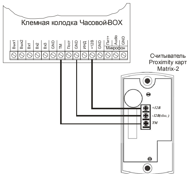
4. Схема подключения различных считывателей ключей.
