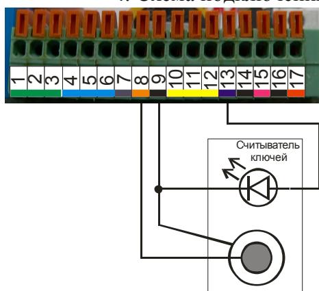
4. Схема подключения различных считывателей ключей.
