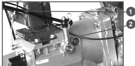
Рис. 12 Коробка передач мотоблока 1. Рычаг переключения передач 2. Тяга переключения
