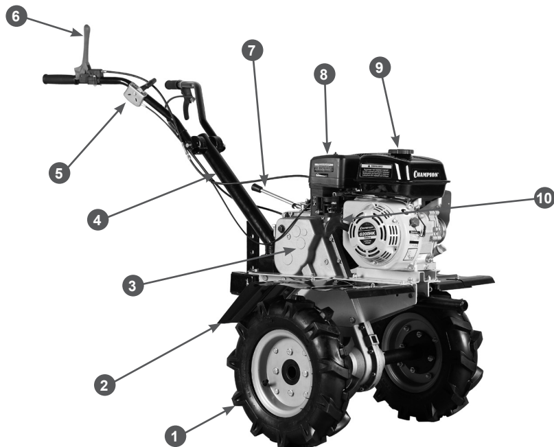
Рис. 1 Основные узлы и органы управления (вид справа)
