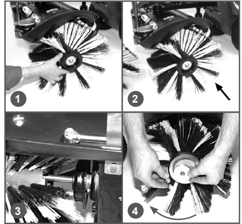
Рис. 5 Установка щеток
