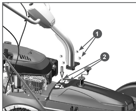
Рис. 2 Установка рукоятки
