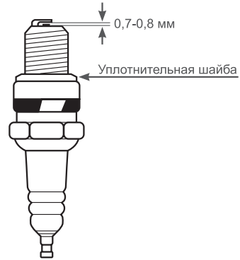
Рис.21 Обслуживание свечи зажигания.
