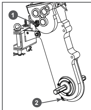
Рис. 38 Замена масла в редукторе
