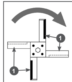
Рис. 5 Расположение ножей на фланцах оси фрезы
