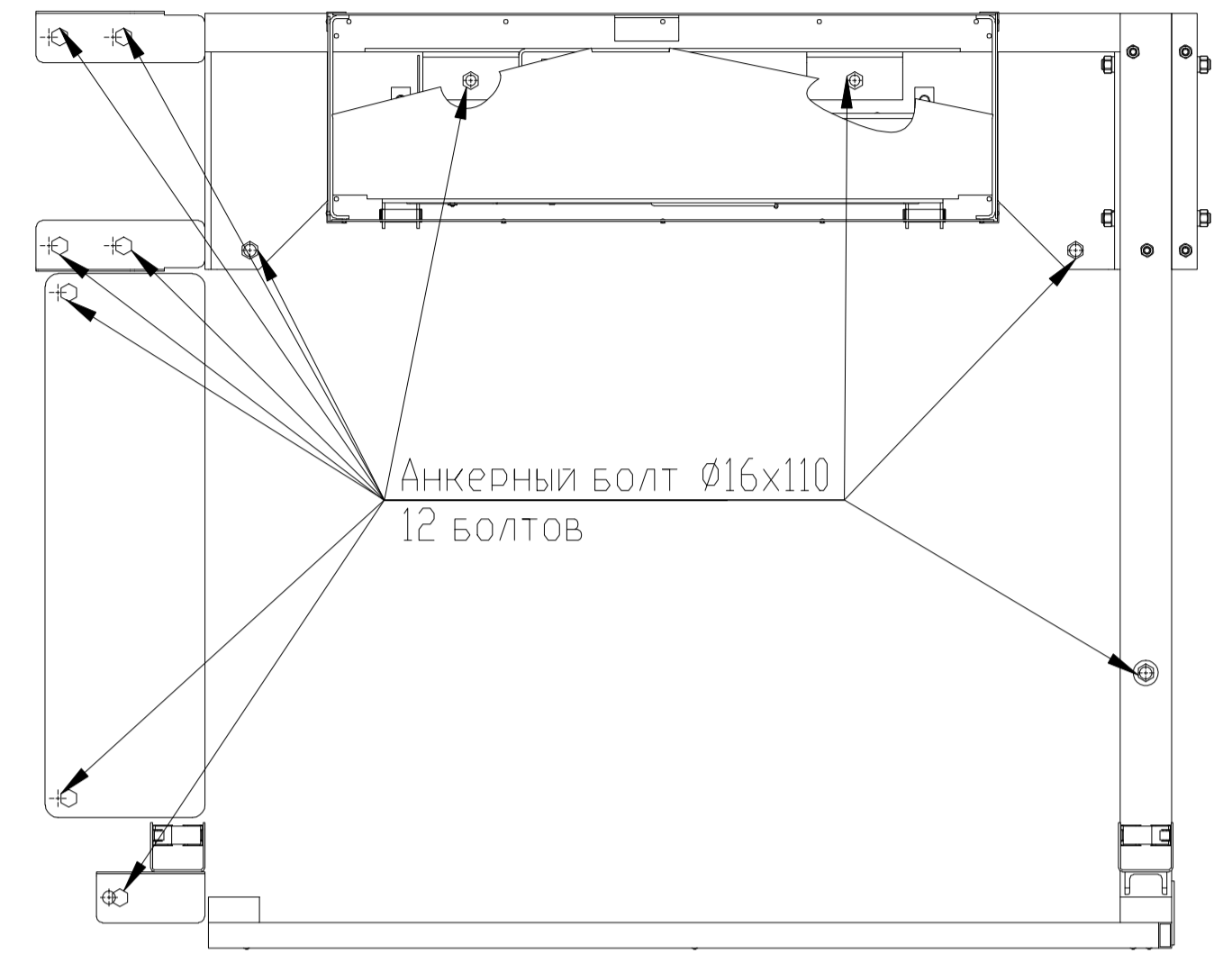
Расположение анкерных болтов
