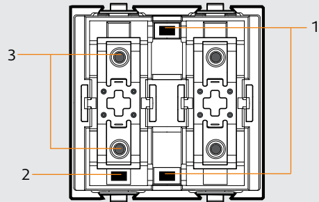
Вид спереди арт. H4574*
