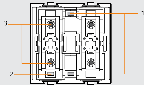
Вид спереди арт. H4573/2*
