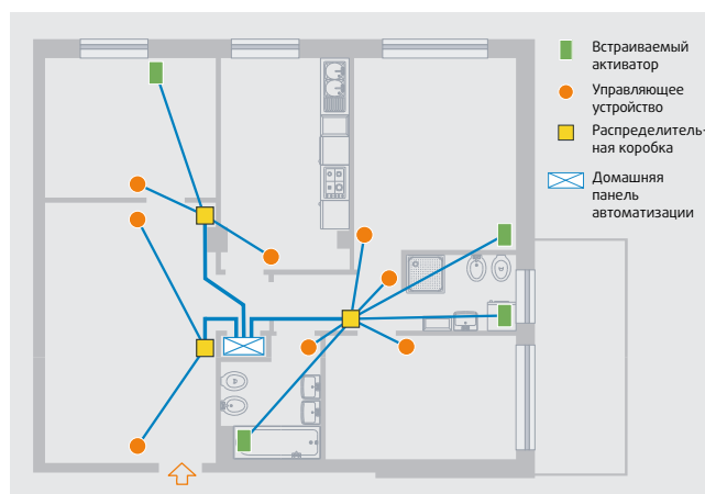
Структура типа «звезда»
