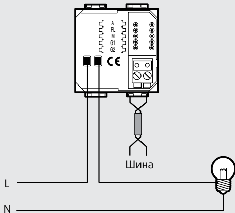
Активатор арт. L4671/1
