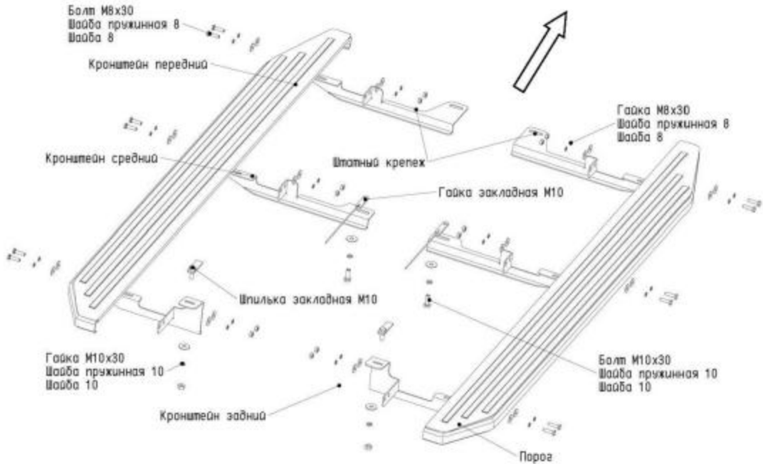
Рис. 1 Схема установки комплекта порогов
