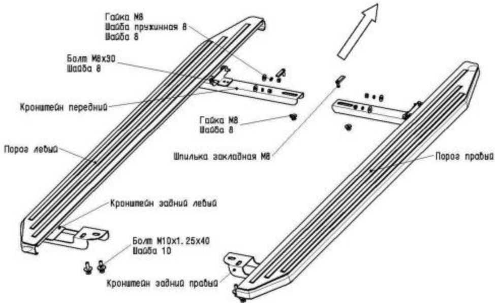
Рис. 1 Схема установки комплекта порогов
