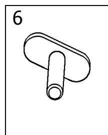
6 Пластина 25x70 со шпилькой М10x35 – 2 шт.
